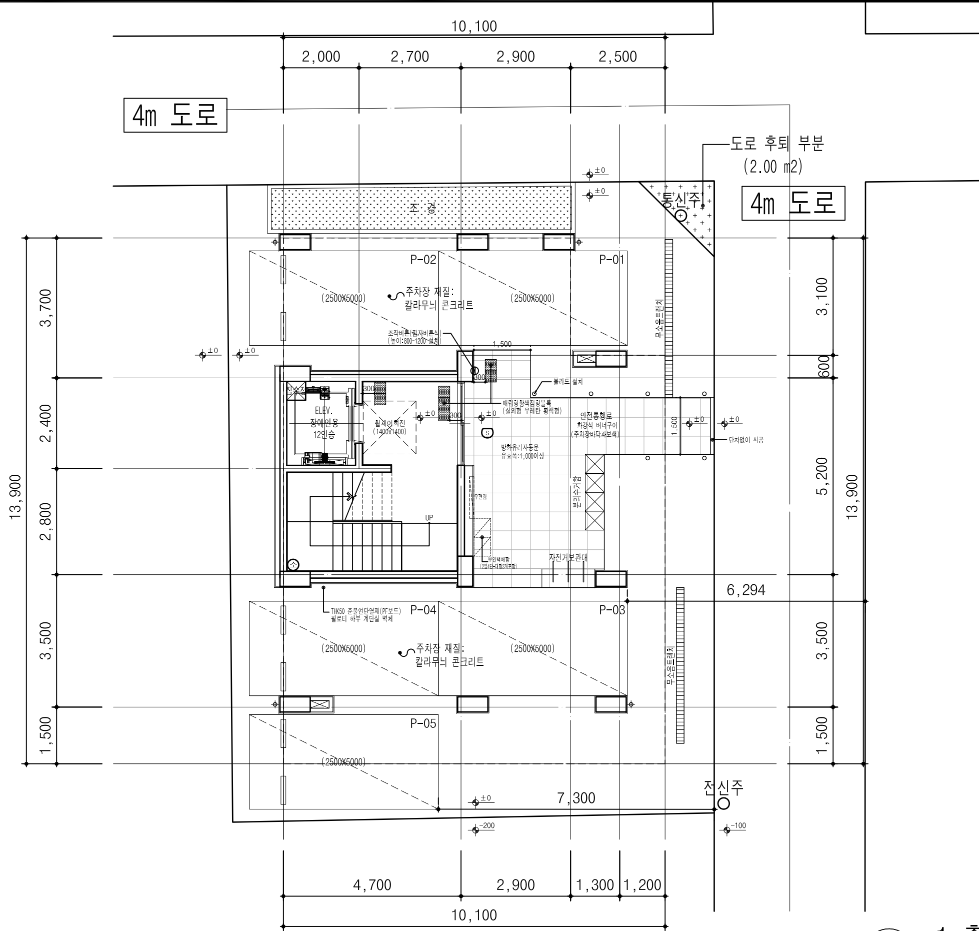
1층 평면도 SCALE : A3 : 1/100
