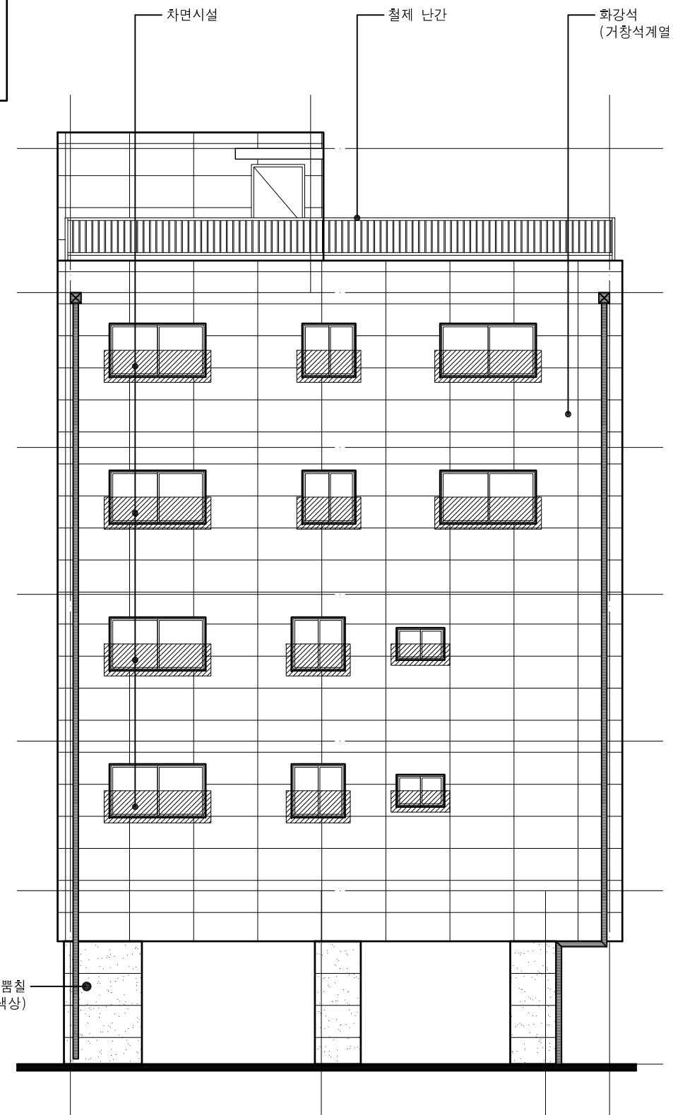
좌 측 면 도 SCALE : A3 : 1/100
