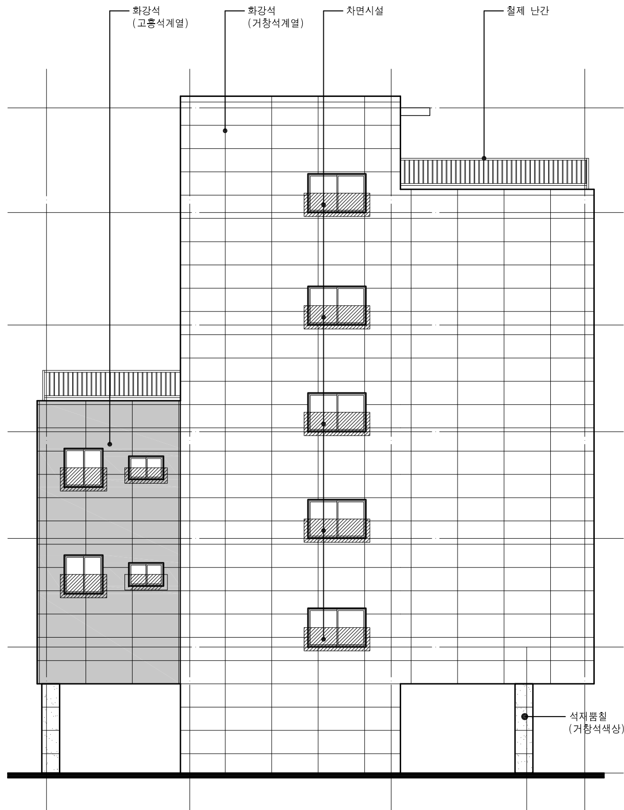
배 면 도 SCALE : A3 : 1/100
